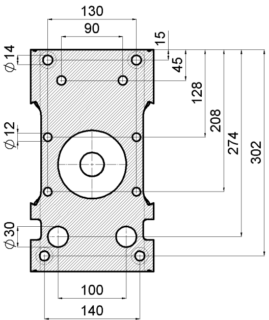
Schnittansicht A-A Bohrbild
